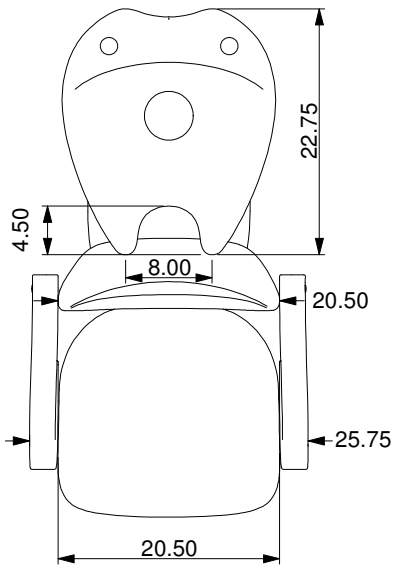
Top
